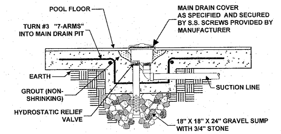
MAIN DRAIN DETAIL N.T.S.
