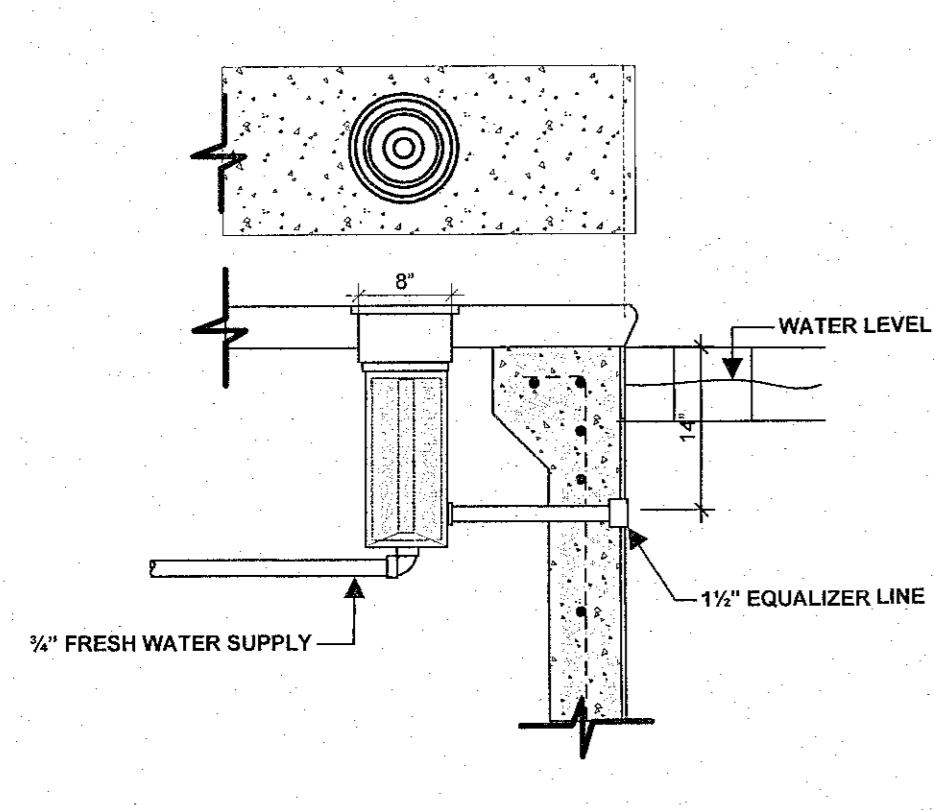
AUTOMATIC FILL DETAIL N.T.S.
