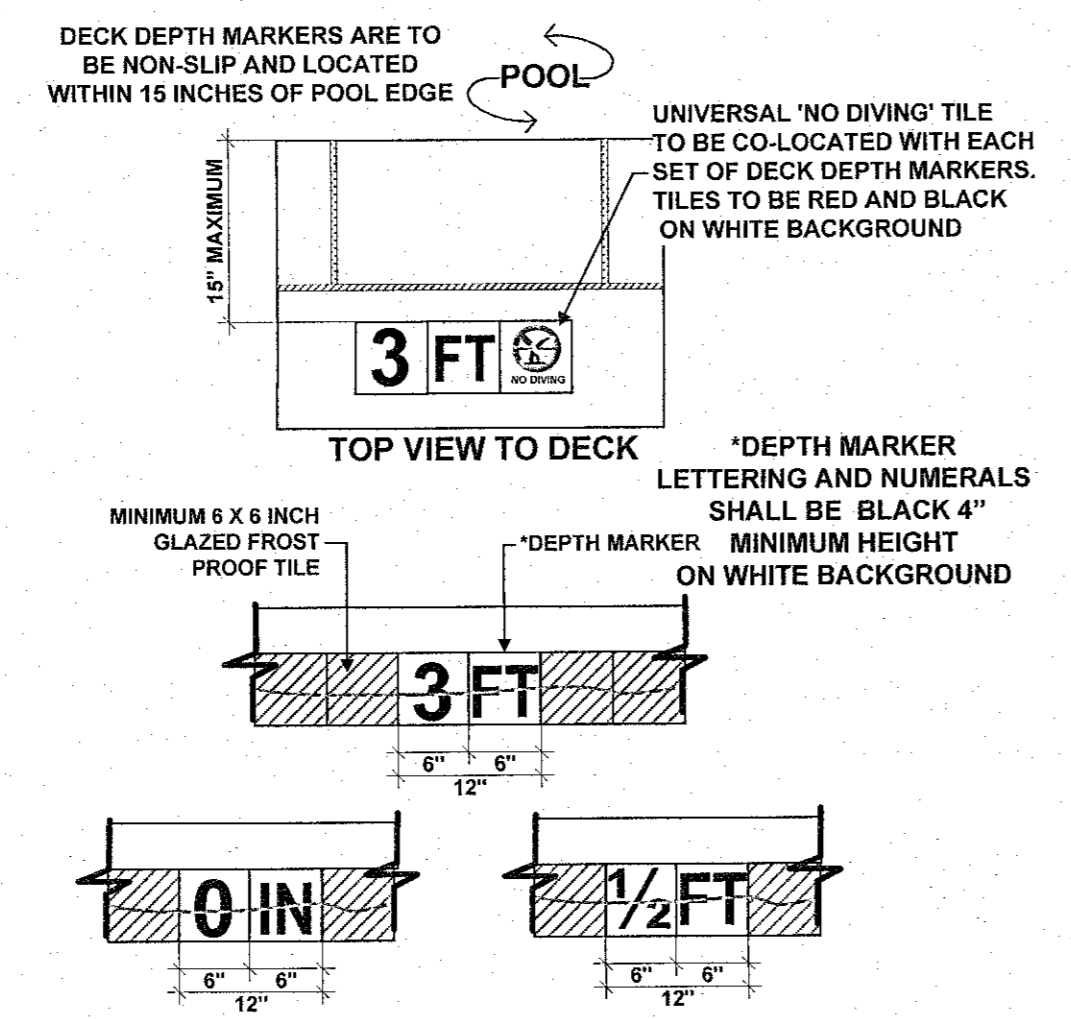
DEPTH MARKER DETAIL N.T.S.
