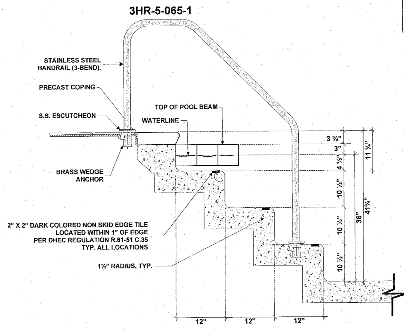
POOL STEP DETAIL N.T.S.
